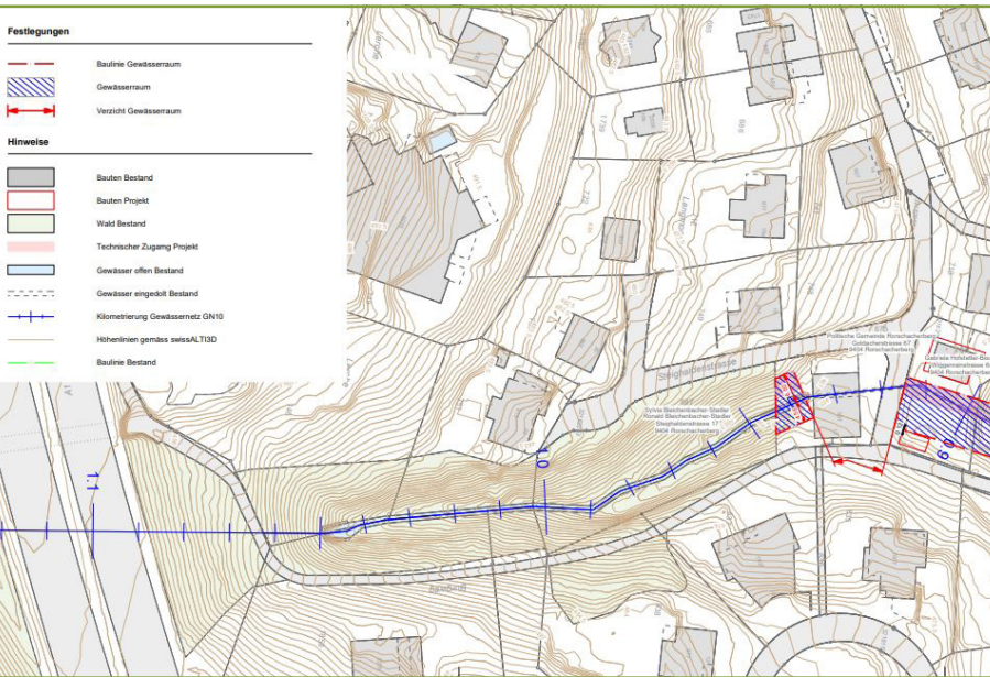
Ausschnitt aus dem Sondernutzungsplan Burgbach
