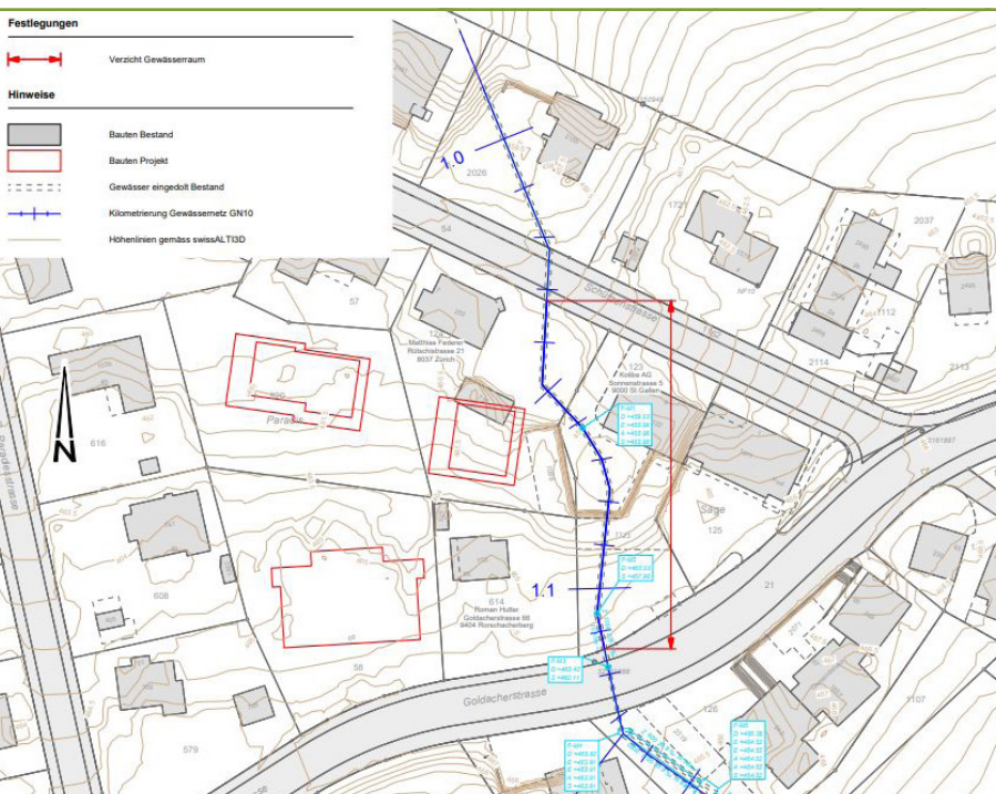
Ausschnitt aus dem Sondernutzungsplan Haiderbach
